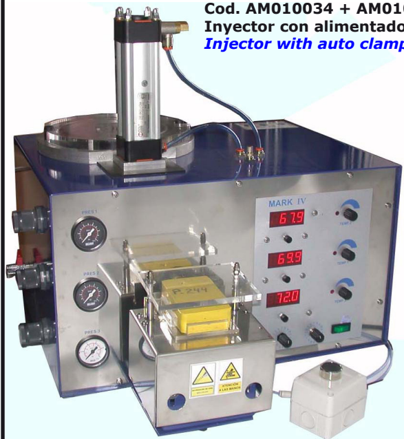
ALIMENTADOR - AUTOCLAMP Cod. AM010034A
