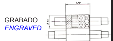
Cod. FD011250 Mod. TD-180 2 Velocidades 2 Speeds
