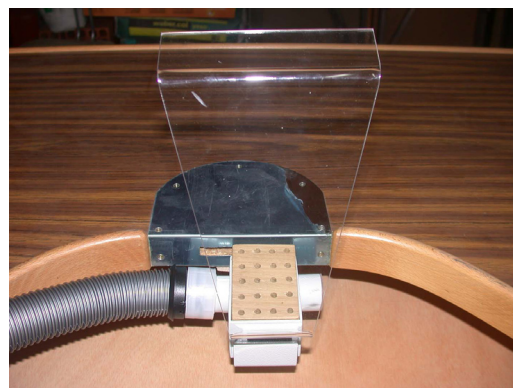
COD. HH016400 Astillera aspiracion.
