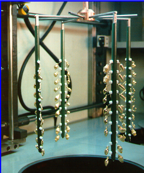
BASTIDOR TIPO V - RACK TYPE V
