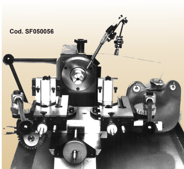
Vista frontal con accesorios para medallas y pulverizador con compresor. Front view with accessories for medals and sprayer with compressor.
