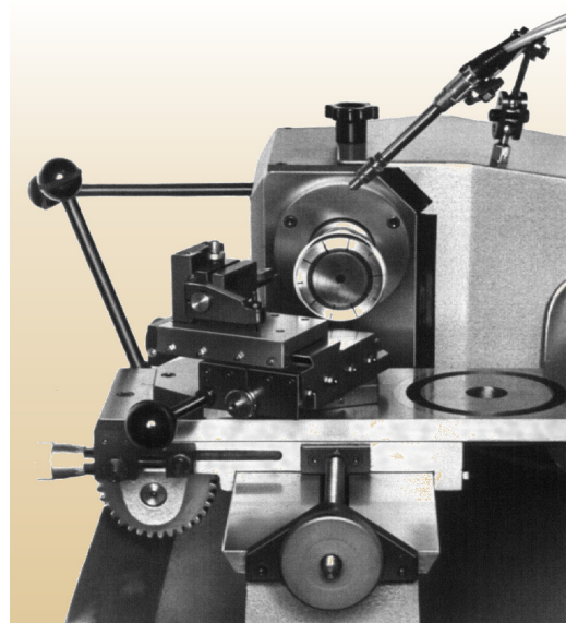
Con utillaje punto redondo (cod. SF050406) y accesorios para facetar brazaletes.
