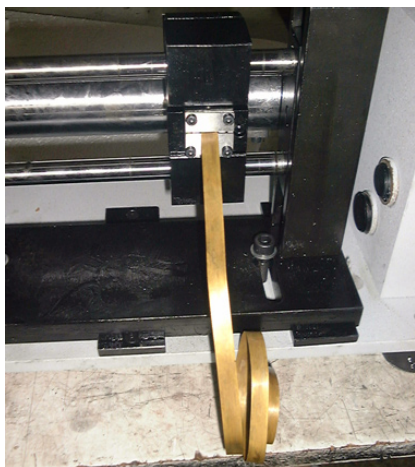
Detalle alimentación fleje Detail strip feeding
